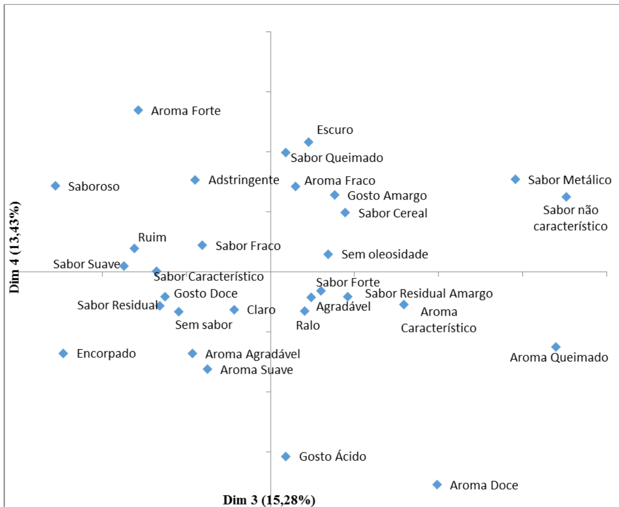
Figura 2 Representação das amostras dos termos na terceira e quarta dimensões da Análise Múltipla de Fatores (MFA) sobre os dados do posicionamento sensorial polarizado.
