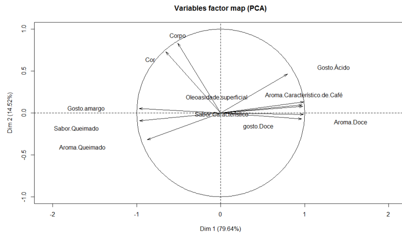
Figura4 Representação das amostras e dos atributos pela Análise de Componentes Principais (ACP) obtida através da análise descritiva com avaliadores treinados
