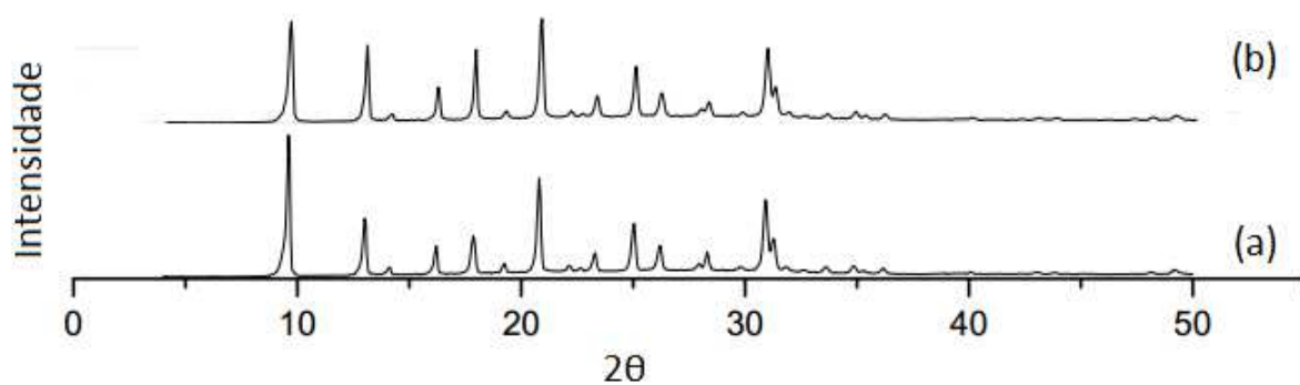
Figura 17 Difratoograma de raios-X das amostras de SAPO-34 com SAR 1,3 e diferentes tempos de reação. (a) 24h; (b) 120h.
