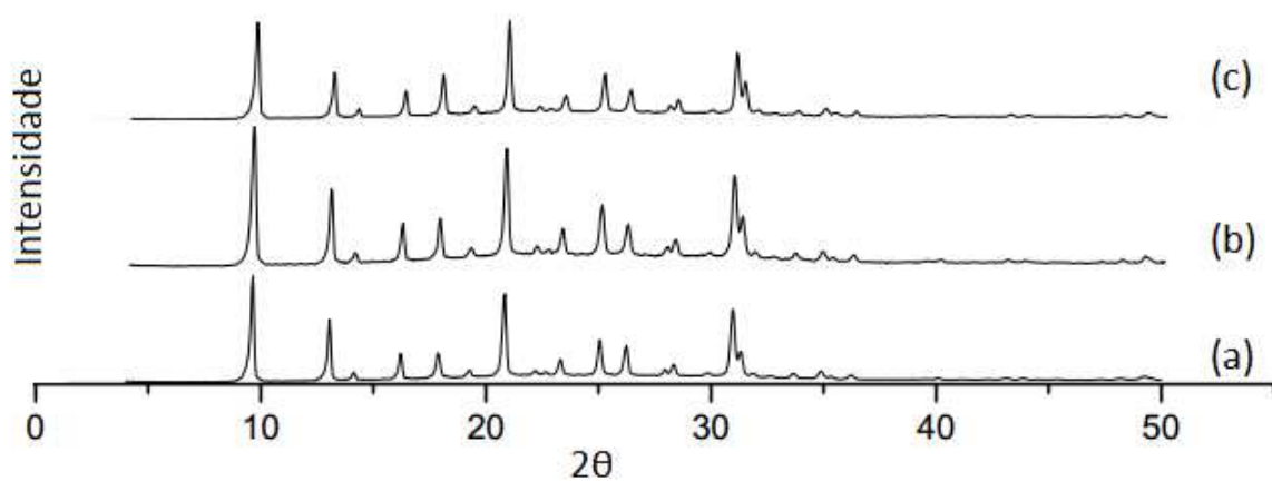
Figura 19 Difratoograma de raios-X das amostras de SAPO-34 com SAR 2,0 e diferentes tempos de reação. (a) 24h; (b) 48h e (c) 120h
