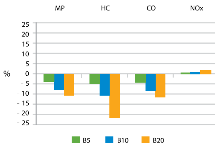
Figura 1: Efeito da adição de biodiesel nas emissões diretas de motores de ciclo diesel (Adaptado de SZULCZYK e McCARL, 2010)
