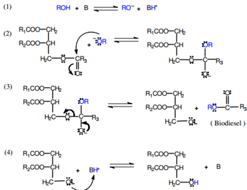
Figura 5: Mecanismo de transesterificação alcalina de óleos vegetais (MA e HANNA, 1999).
