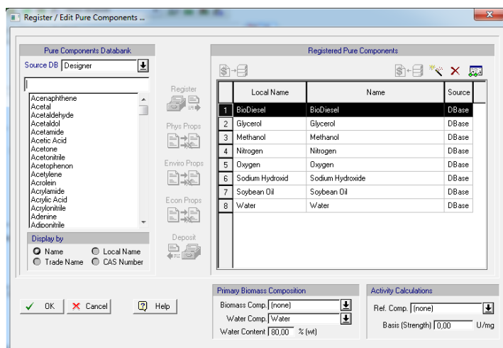
Figura 18: Interface do registro dos componentes presentes na base de dados do simulador.
