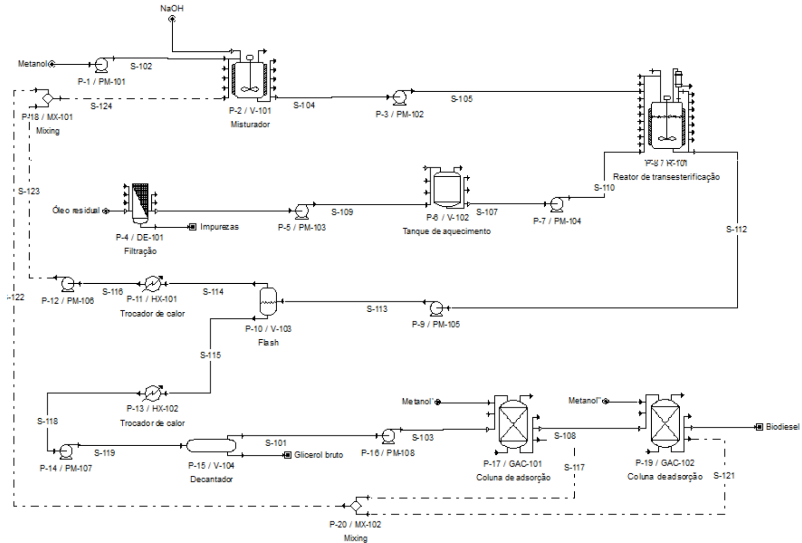
Figura 20: Fluxograma da produção de biodiesel por transesterificação alcalina homogênea
