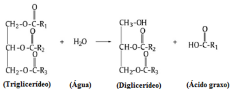
Figura 7: Reação de hidrólise de triglicerídeos
